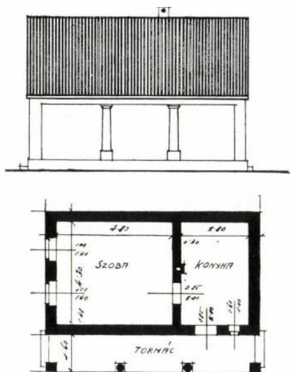
A legkisebb lakóházegység terve Peregén.
